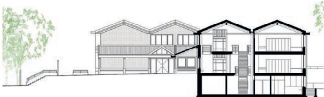
Schnitt Anbau Imbach II
